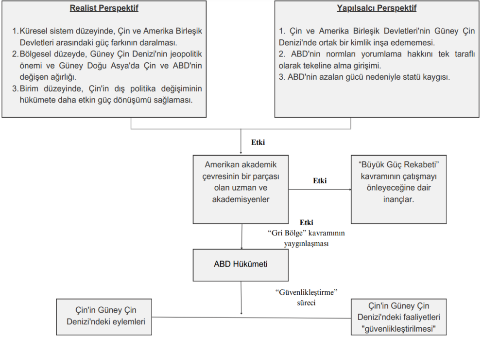
Şekil 8. "Gri Bölge" kavramının yayılmasının, ABD'nin Güney Çin Denizi sorununa müdahil olma sürecine etkisi
