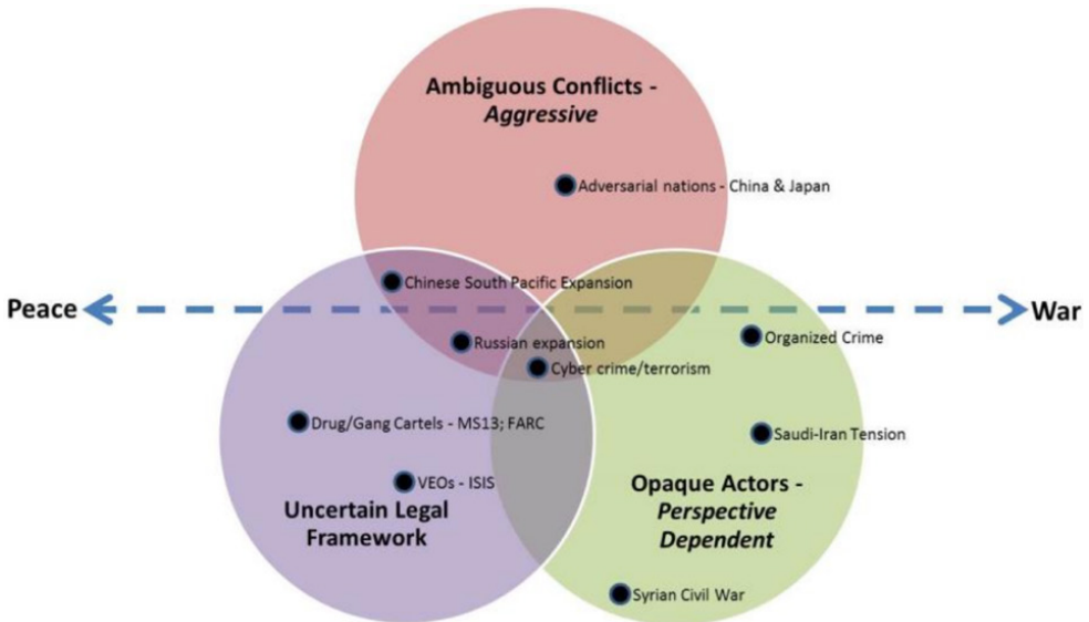
Şekil 4. Gri Bölge Karakteristiği (United States Special Operations Command, 2016)
