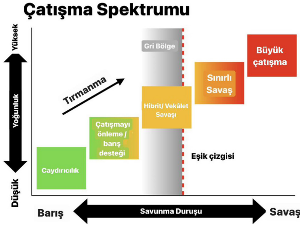
Şekil 3. Gri Bölge Çatışma Spektrumu
