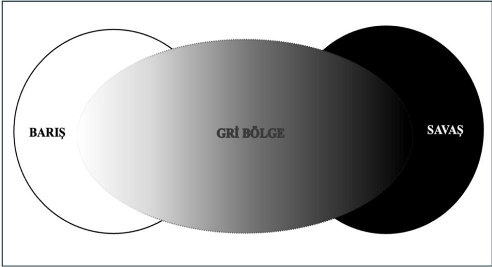
Şekil 1. Gri Bölgenin Savaş ve Barış Arasındaki Kesişimi
